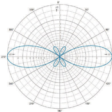
E-Plane | 445 MHz
