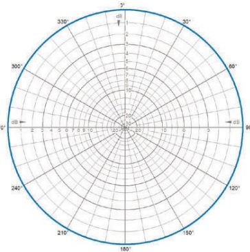
H-Plane | 445 MHz
